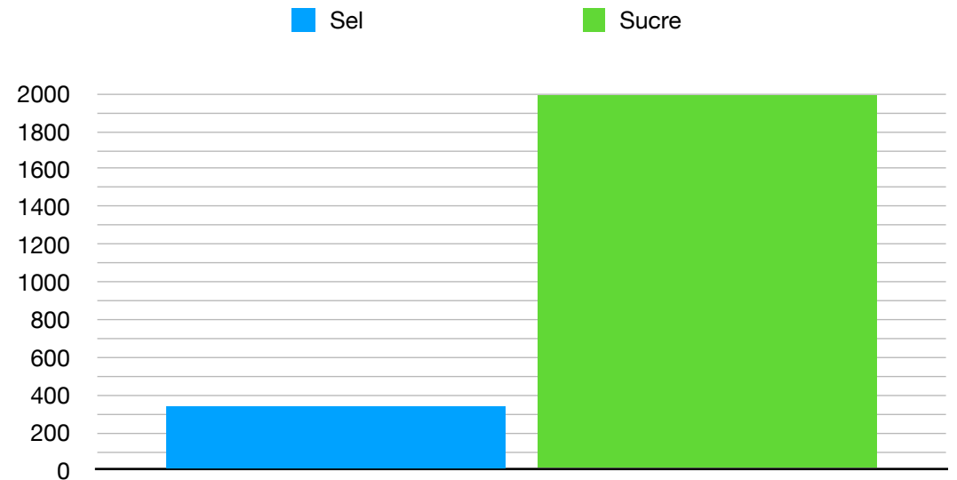
Document 3: La solubilité du sel et du sucre en gramme par litre (g/L)
